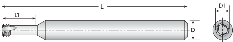
Левая фреза, вращение против часовой стрелки
