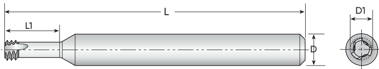
Левая фреза, вращение против часовой стрелки
